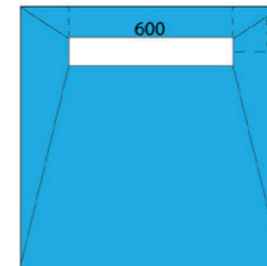
UT PDeck 201 LIN 1000 x 1000 x 22mm
