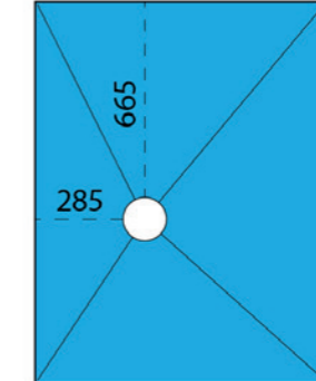
UT PDeck 107 SQ 1135 x 770 x 22mm
