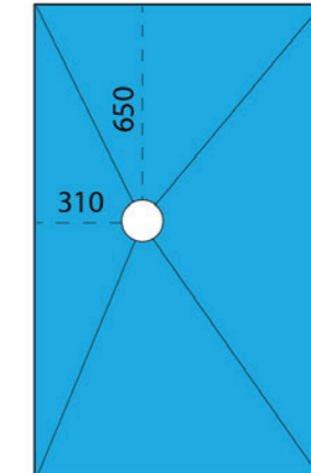
UT PDeck 111 SQ 1500 x 800 x 22mm
